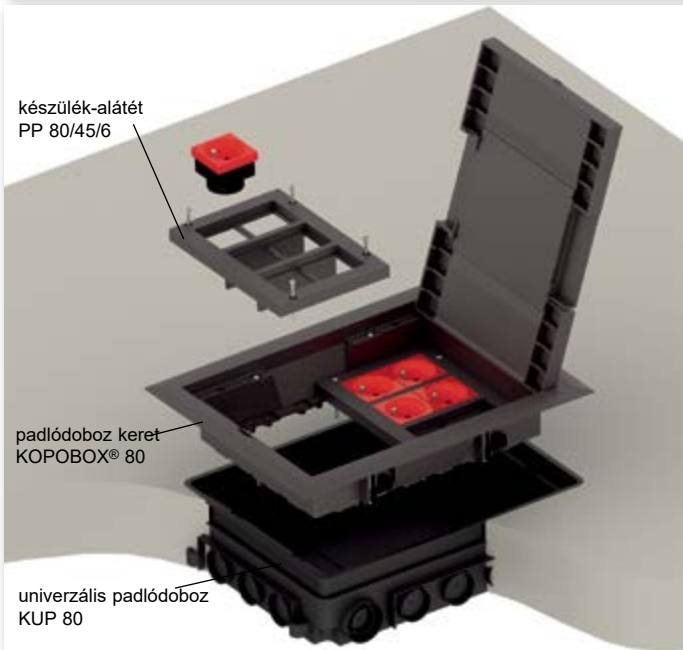
univerzális padlódoboz KUP 80
